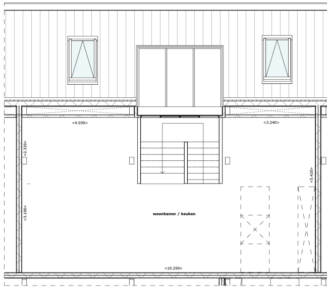
Plattegrond verdieping 04 1:50
